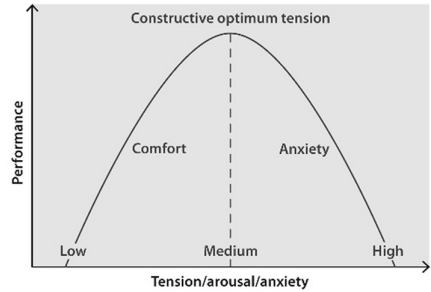
Fig. 5.1.1: Yerkes–Dodson curve.
